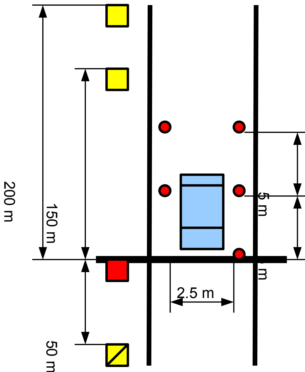
rys. nr 1 Schemat próby Stop Start
